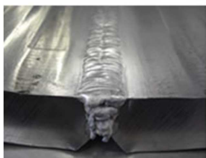
極厚板アルミパイプ A5052 t45 口径φ900×800L
